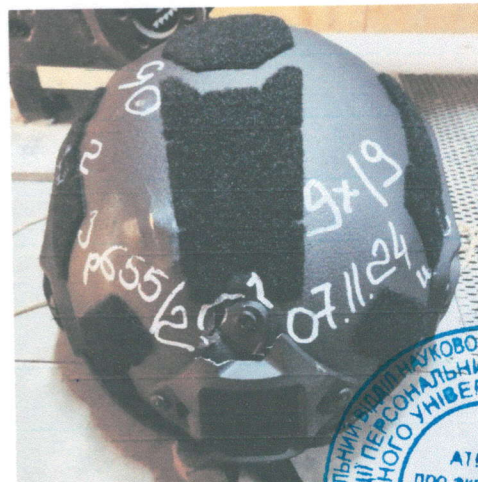
Фото 2 (зразок 655/2 після випробувань)
